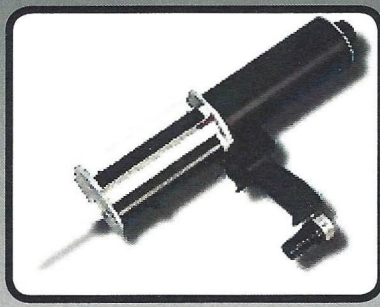
400-мл пневматический нагнетатель № OCR LL005
